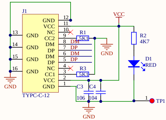
TYPE-C接口电路
